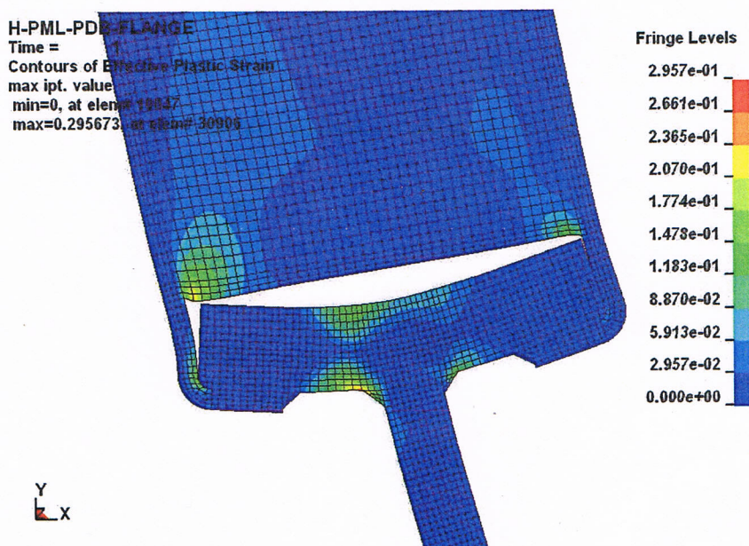
Figuur 1: Effective strain in het 2D eindige elementen model.
