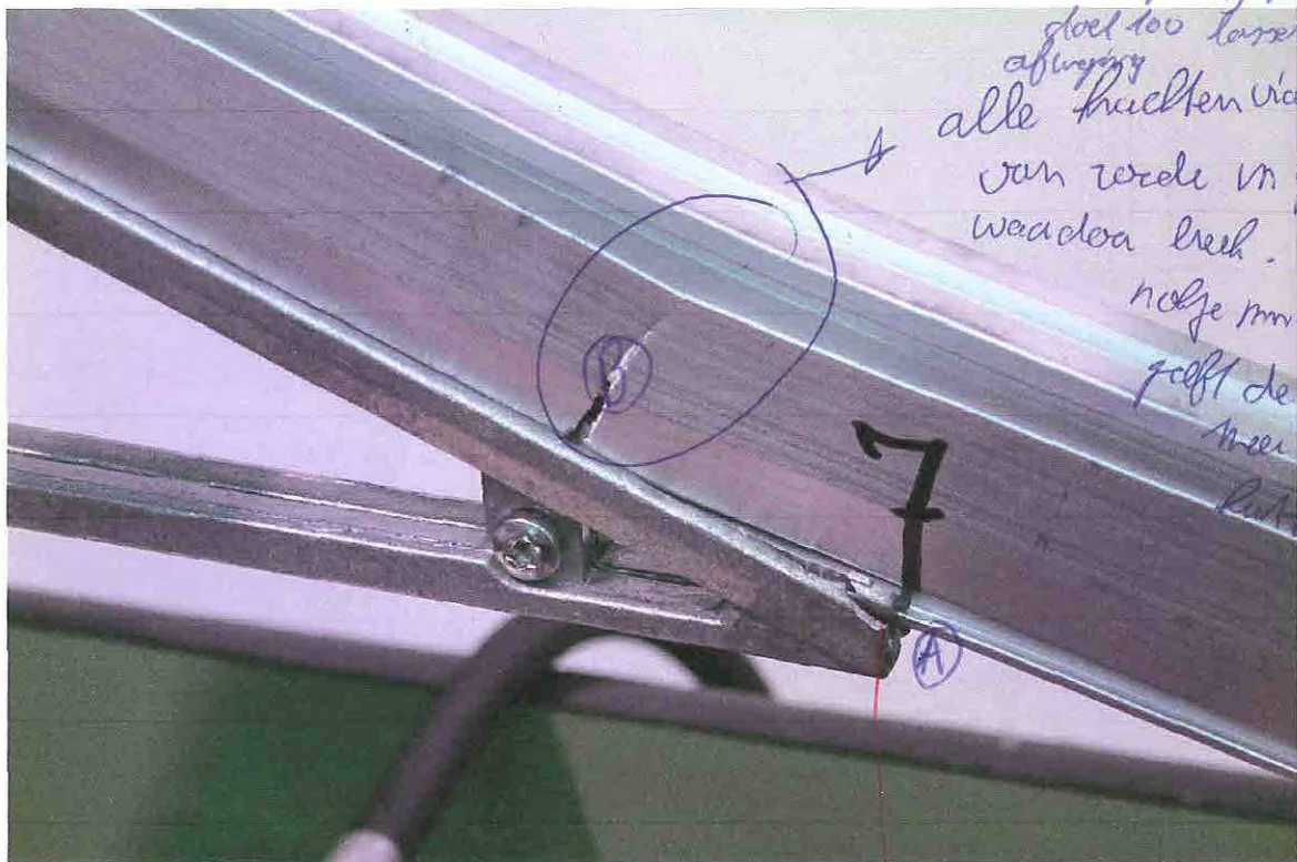
Bezwijkvorm bij simulatie van opwaartse (wind)belasting
